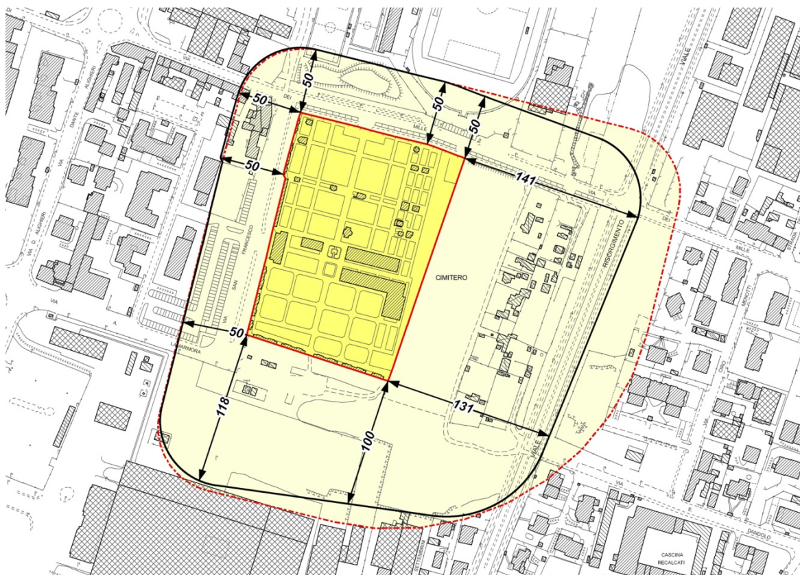
Schema ridefinizione area di rispetto cimiteriale
