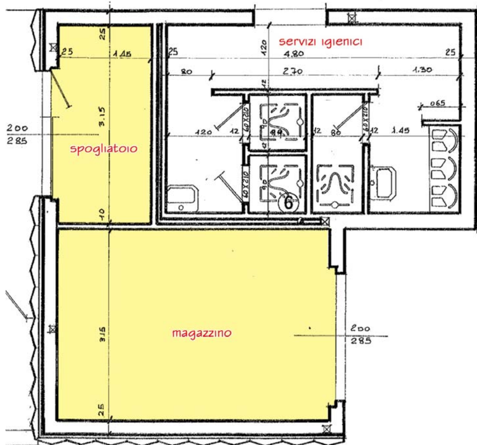
Pianta locali magazzino e spogliatoio
