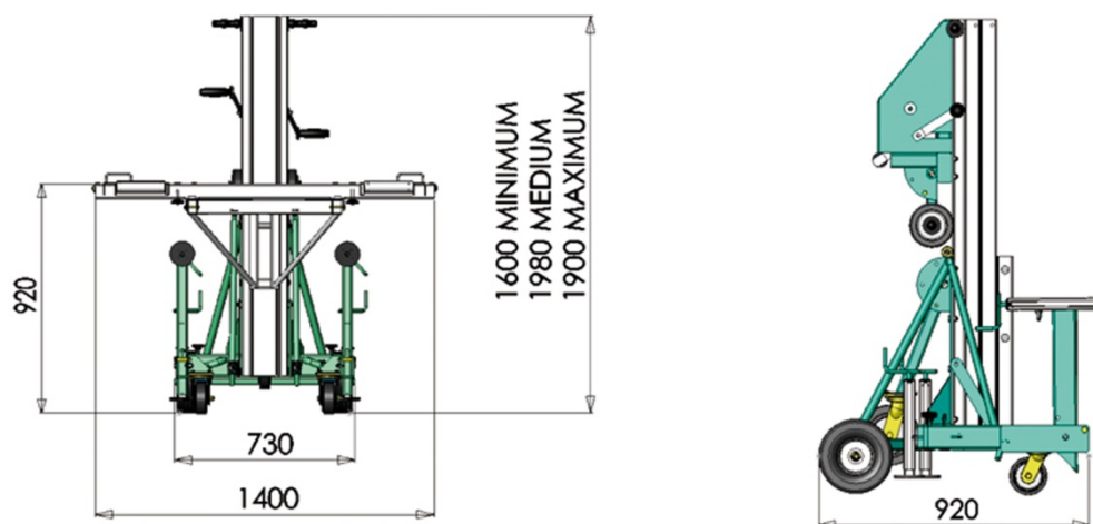
Schema dimensionale di un alzaferetri tipo
