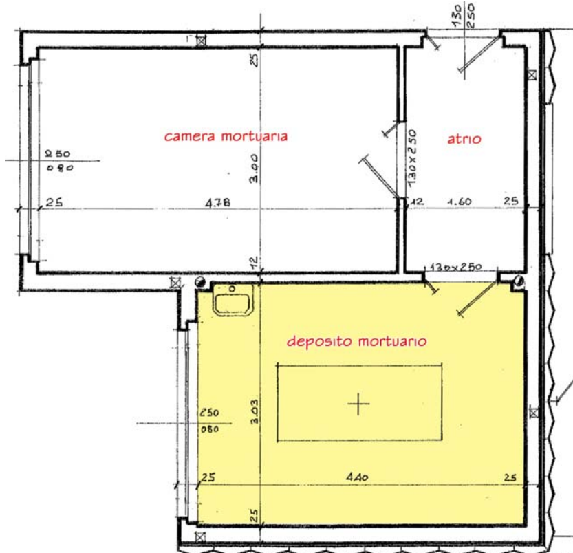
Pianta deposito mortuario
