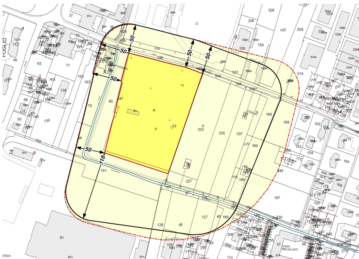
Schema ridefinizione area di rispetto cimiteriale su base catastale
