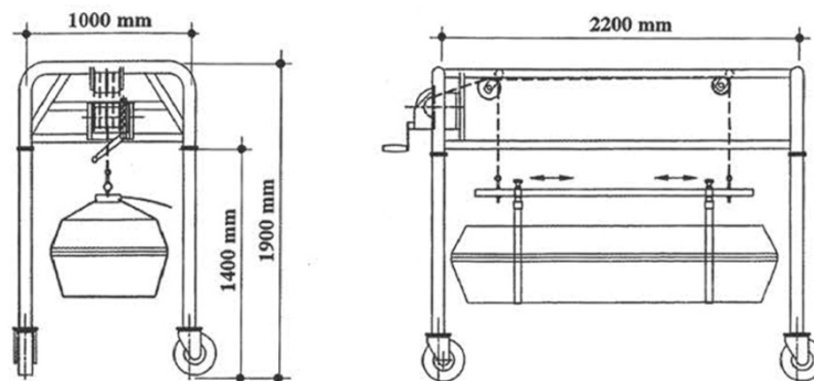
Schema dimensionale di un calaferetri tipo
