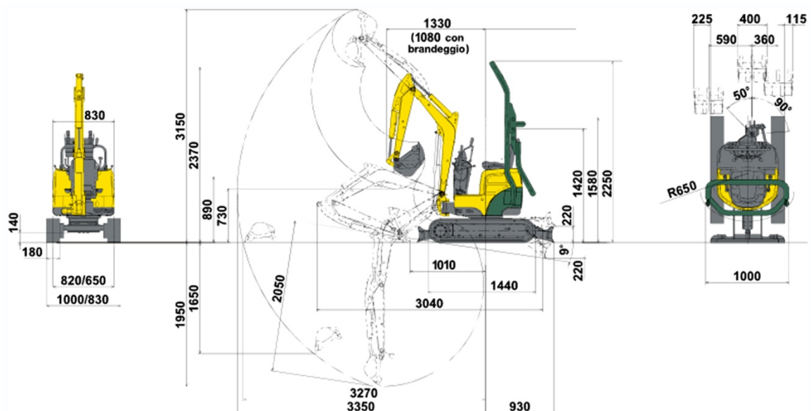
Schema dimensionale di un miniescavatore tipo
