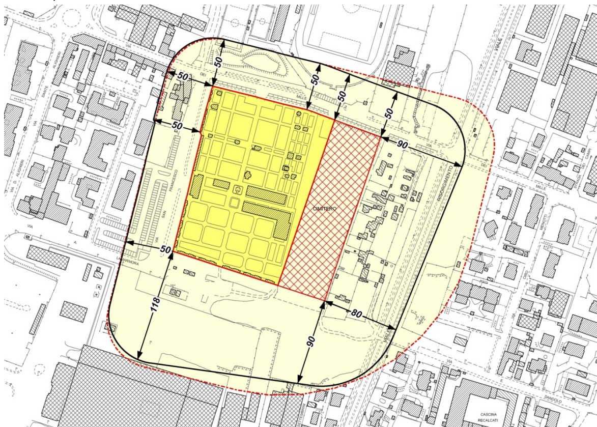
Schema area di ampliamento cimiteriale con distanza fascia di rispetto cimiteriale ridefinita
