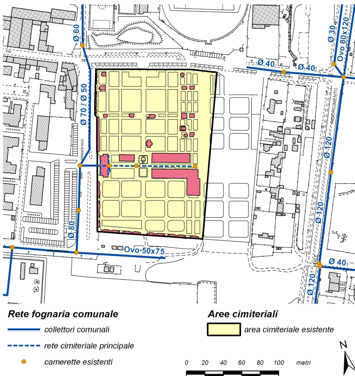
Schema rete fognaria esistente
